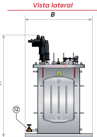
Vista posterior
